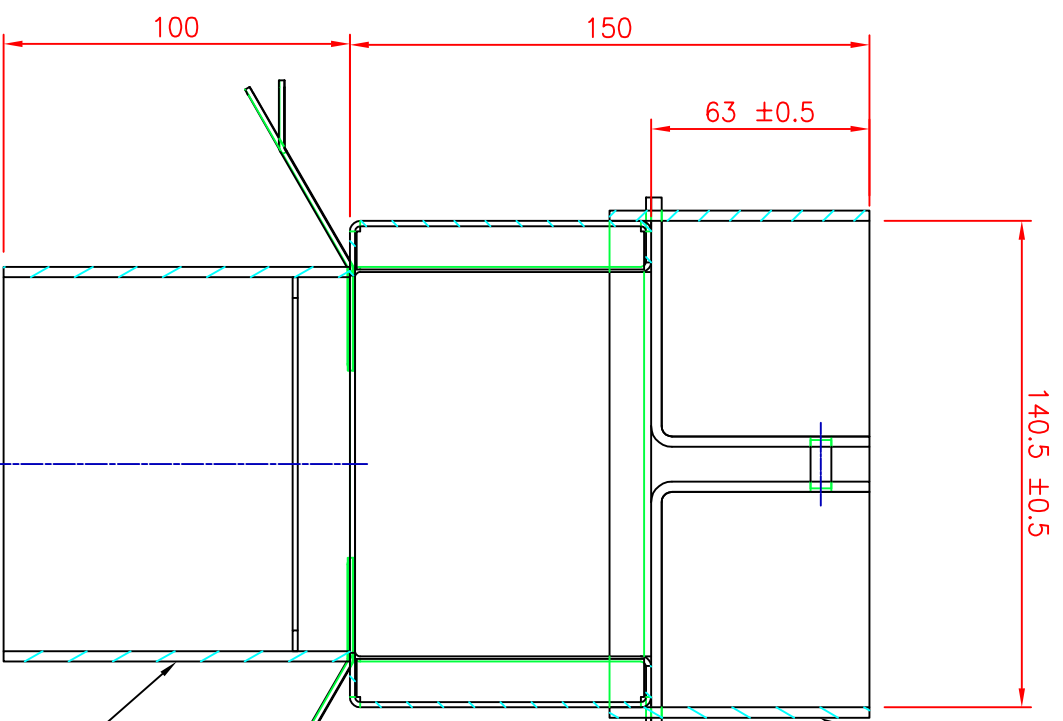
A-A (1:2)
