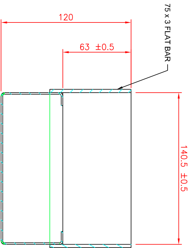
C-C (1:2)
